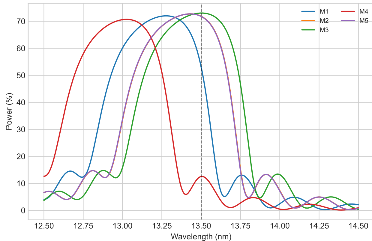
Reflectivity of each Ru/Mo-Si mirror
